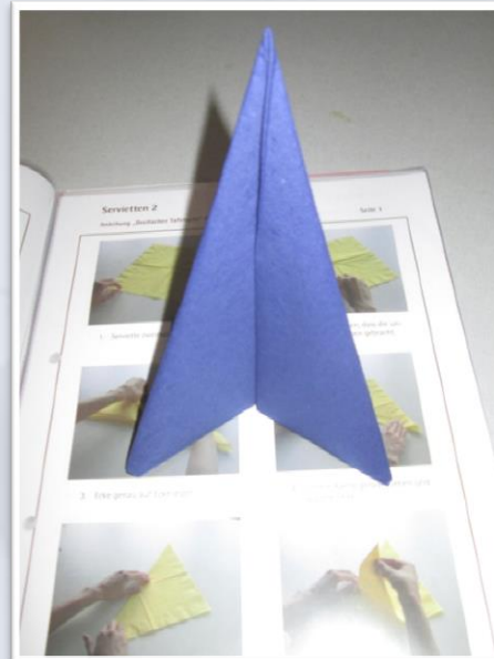
Складывание салфетки
