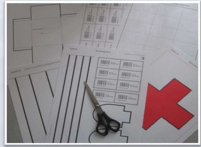
Вырезание ножницами
